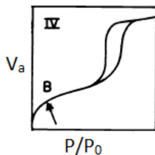
شکل ۱۰- ایزوترم جذب نوع IV [13].
