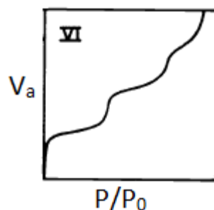
شکل ۱۲- ایزوترم جذب نوع VI [13].
