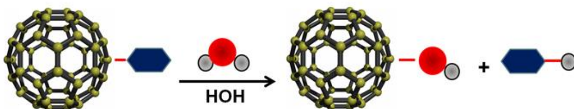
شکل ۲- شمایی از آب کافت مولکول فولرن ( \text{C}_{60} ).
