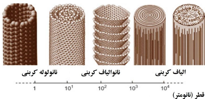
شکل ۹- شمایی از ساختار و ابعاد الیاف، نانوالیاف و نانولوله‌های کربنی [1].
