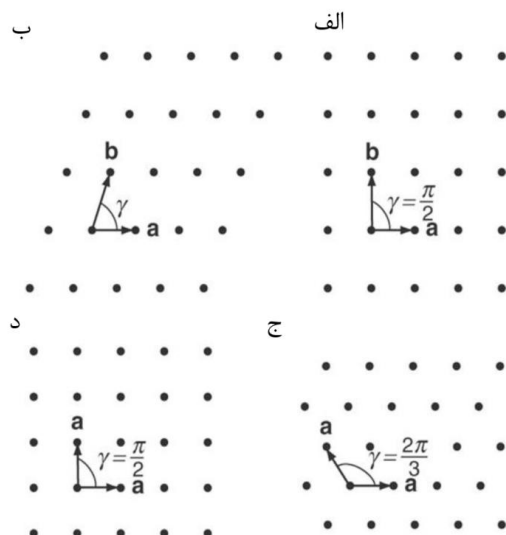
شکل ۲- چهار سیستم بلوری مختلف در دوبعد (الف) سیستم مستطیلی (ب) مورب ۹ (ج) شش ضلعی (د) مربعی [۱]
