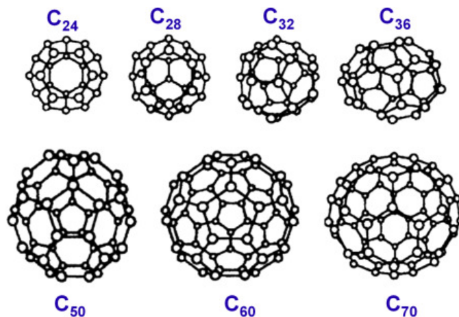
شکل ۱۱- شمایی از شبکه بلوری هم‌پارهای فولرین با تعداد کربن مختلف [2].
