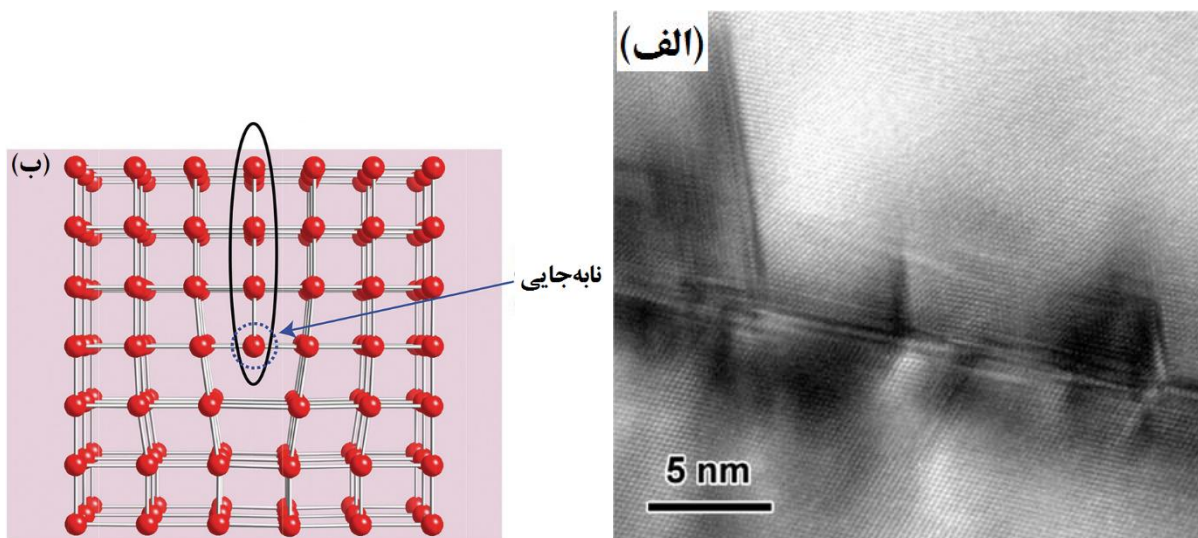
شکل ۲- (الف) تصویر میکروسکوپ الکترونی عبوری (TEM) و (ب) شمایی از نقص نابه جایی [1].
