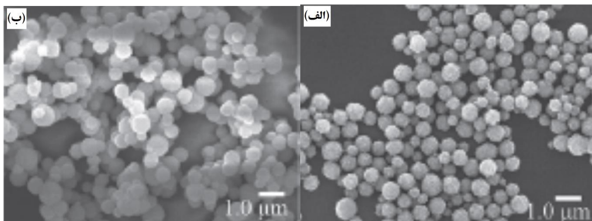
شکل ۱- تصویر میکروسکوپ الکترونی روبشی (SEM) از مورفولوژی نانوذرات تیتانیوم دی اکسید سنتز شده با روش ترسیب شیمیایی همگن در دماهای (الف) ۸۰ و (ب) ۱۰۰ درجه سانتی گراد [1].
