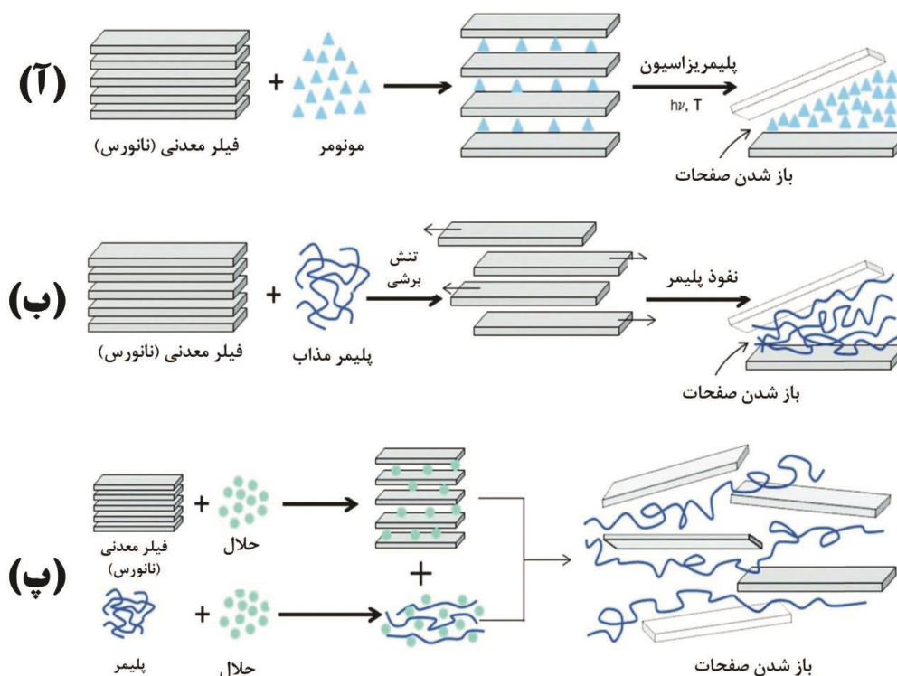
شکل ۴: تصویر شماتیک از روش های ساخت نانو کامپوزیت زمینه پلیمری و نانوصفحات رسی (آ) روش پلیمریزاسیون درجا، (ب) روش اختلاط مذاب، (پ) روش حلالی [۳]
