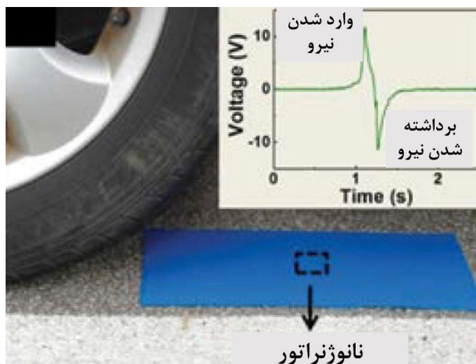
شکل ۸- استفاده از نانوسیم های اکسید روی به عنوان نانوژنراتور برای تولید الکتریسیته از حرکت خودروها بر روی صفحه نانوژنراتور
