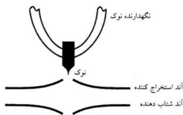
شکل ۲- خروج الکترون از نوک فلز و هدایت آن به وسیله آند استخراج کننده و شتابدار نمودن آن به وسیله آند شتاب دهنده
