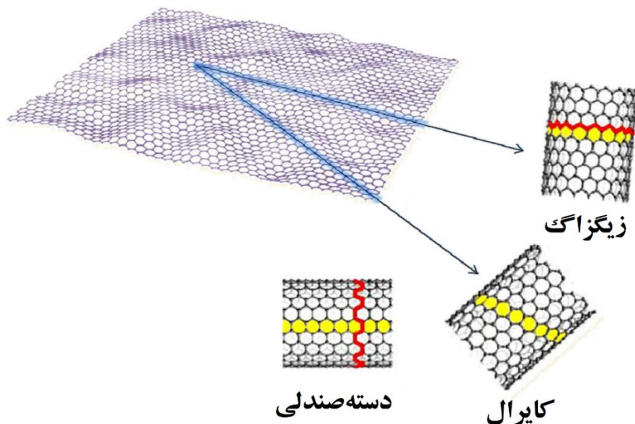
شکل ۳- شمایی از سه گروه مختلف نانولوله های کربنی برحسب مولفه و زاویه کایرال [2].
