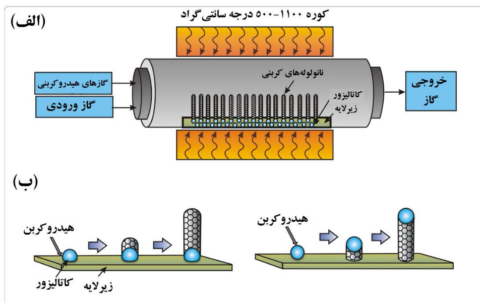
شکل ۶- (الف) شمایی از فرآیند رسوب‌دهی شیمیایی از فاز بخار برای سنتز نانولوله‌های کربنی و (ب) مکانیزم‌های رشد نانولوله‌ها [4].
