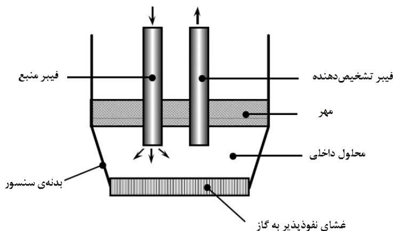
شکل ۳- یوسنسور فیبر نوری [۳]
