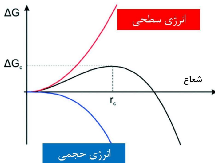
شکل ۳- تغییرات انرژی آزاد با توجه به شعاع هسته ایجاد شده [۲]
