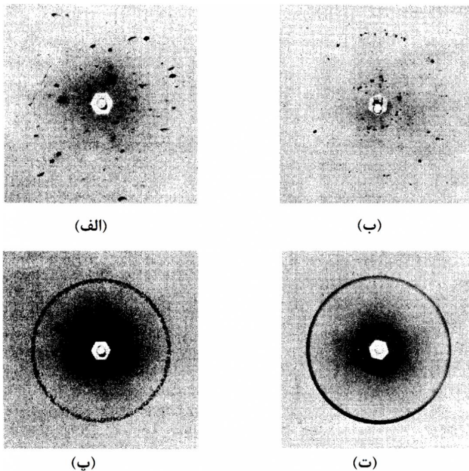
شکل ۲- الگوهای سوراخ پس بازتاب نمونه های آلومینیومی تبلور مجدد یافته؛ اندازه دانه به ترتیب از (الف) تا (ت) کاهش می یابد.
