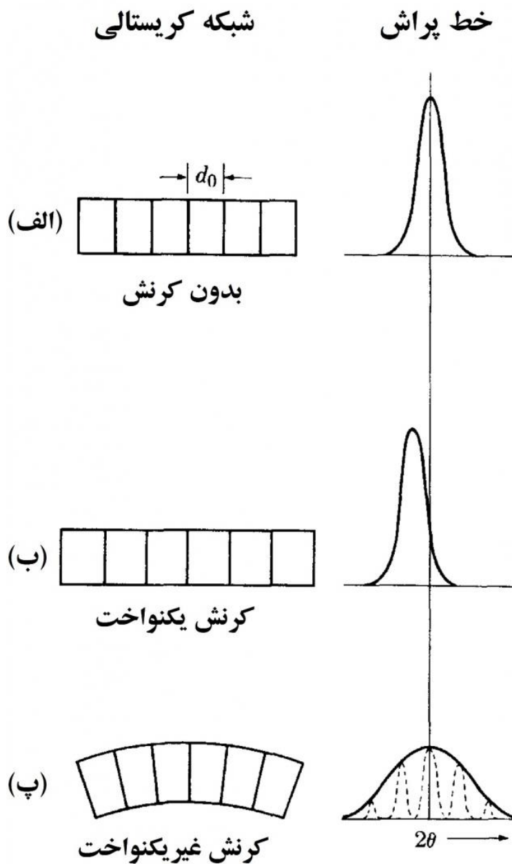
شکل ۶- تاثیر کرنش شبکه روی موقعیت و پهنای خط پراش.
