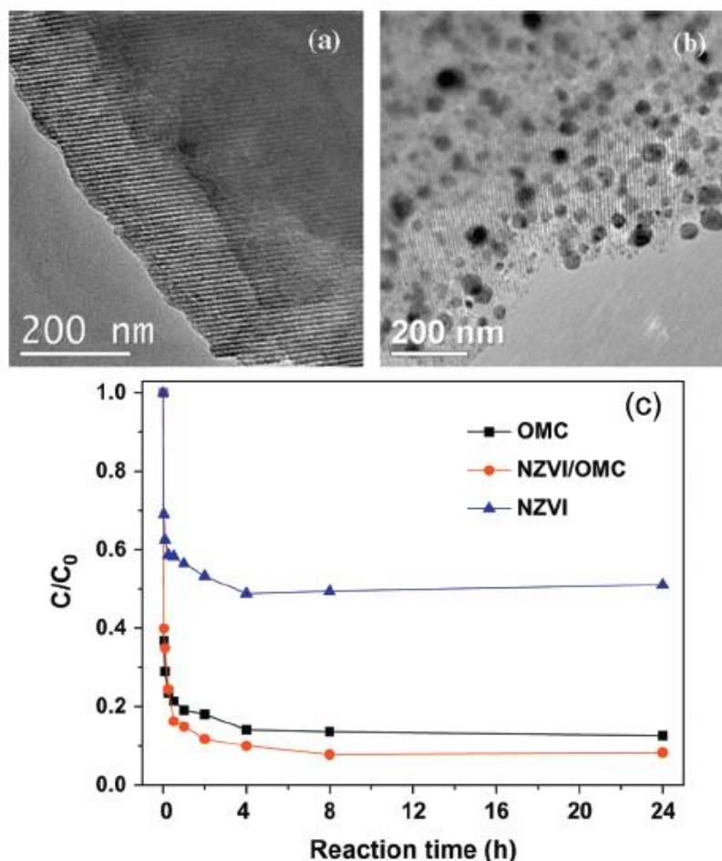
شکل ۲. الف) تصویر میکروسکوپ الکترون عبوری کربن مزومتخلخل و ب) کامپوزیت کربن مزومتخلخل و نانوذرات آهن صفر ظرفیتی پ) نسبت غلظت آلاینده به غلظت اولیه بر حسب زمان برای هر کدام از جاذبها [۲۳]
