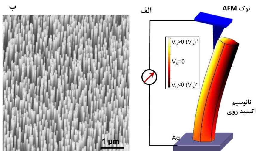
شکل ۴- الف) ایجاد انحنا در نانوسیم اکسیدروی و بررسی انرژی الکتریکی ایجاد شده (ب) نانوسیم‌های اکسیدروی که به صورت موازی بر روی سطح رشد نموده‌اند [۳]
