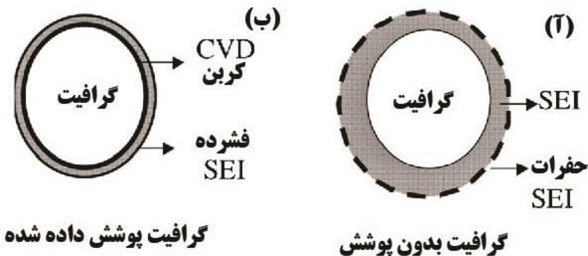
شکل ۵. الف) آند بدون پوشش کربنی ب) آند با پوشش کربنی
