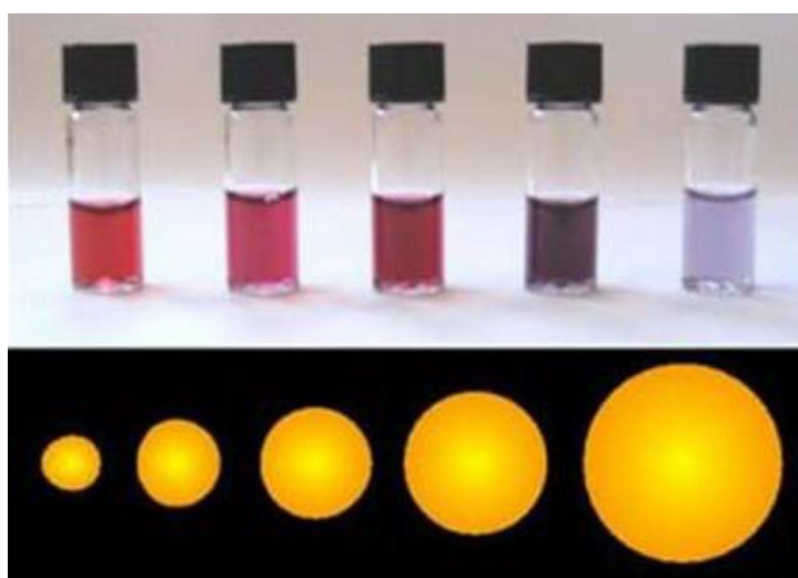
شکل ۱: تغییر رنگ کلویید نانوذرات طلا در اثر افزایش اندازه نانوذرات طلا
