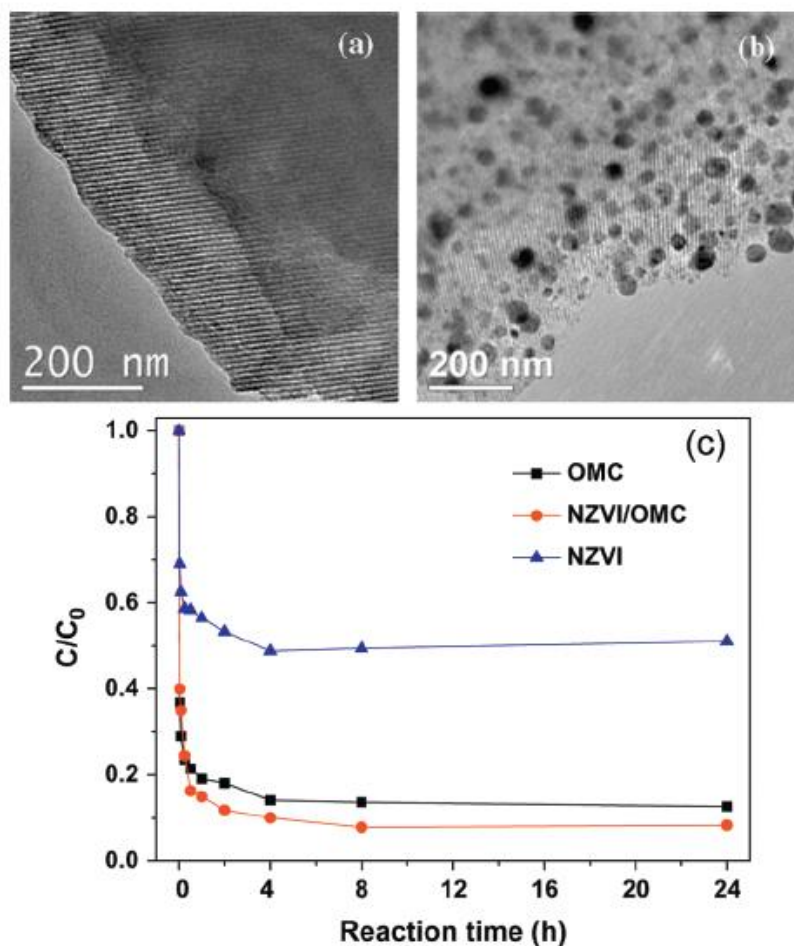
شکل ۲. الف) تصویر میکروسکوپ الکترون عبوری کربن مزومتخلخل و ب) کامپوزیت کربن مزومتخلخل و نانوذرات آهن صفرفیتی (پ) نسبت غلظت آلاینده به غلظت اولیه بر حسب زمان برای هر کدام از جاذبها [۲۳]
