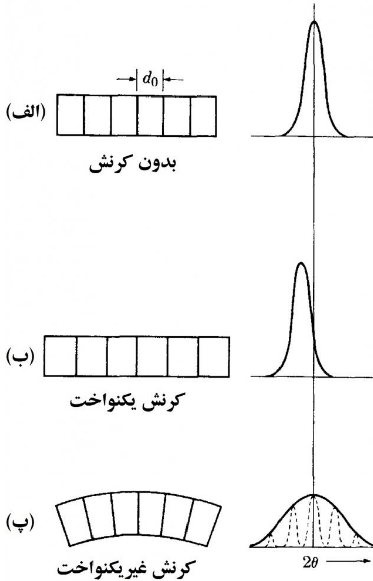
شکل ۶- تاثیر کرنش شبکه روی موقعیت و پهناي خط پراش.
